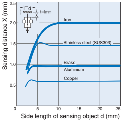
E2A-S08□N02
