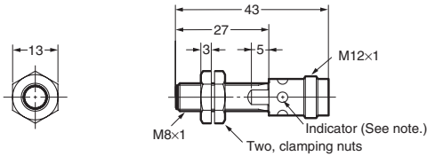
E2A-S08KS01-M1-□□
