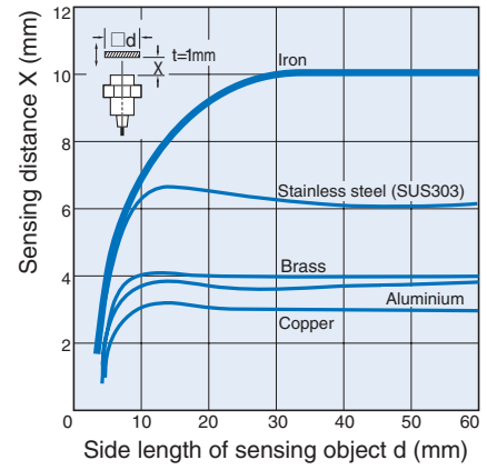
E2A-M18□N10/E2A-S18□N10
