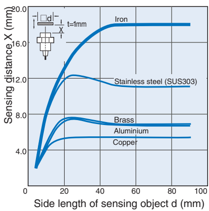
E2A-M30□N18/E2A-S30□N18
