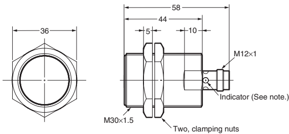
E2A-M30KS10-M1-□□/E2A-S30KS10-M1-□
