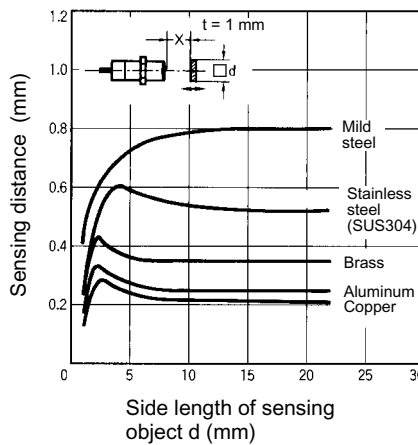
E2E-CR8□□
