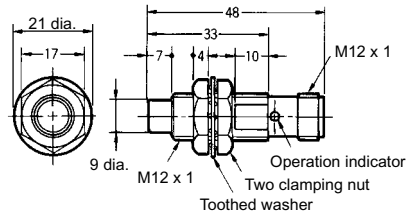
Fig. 22 : E2E-X5MY□-M1
