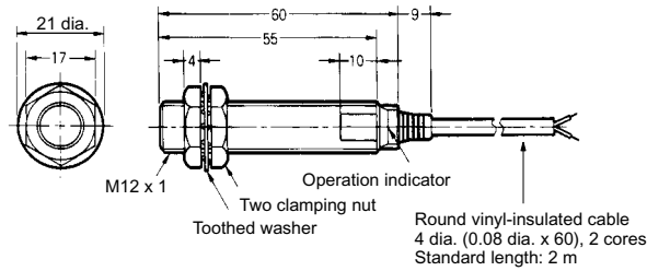
Fig. 13 : E2E-X7D□-N/E2E-X5E□/F□ E2E-X5Y□/E2E-X7T1
