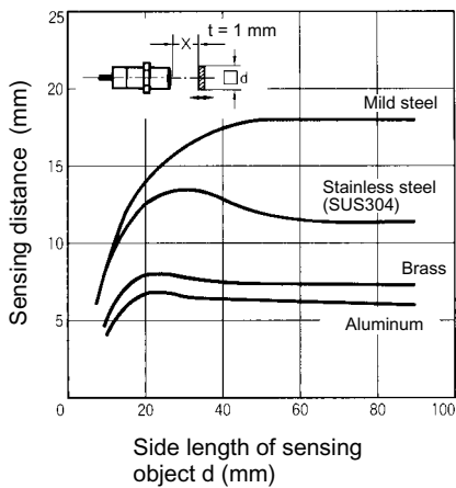
E2E-X18ME□/F□ E2E-X18MY□
