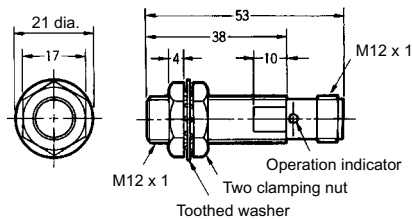
Fig. 23 : E2E-X7D□-M1G/E2E-X5E□-M1/F□-M1 E2E-X5Y1-M1
